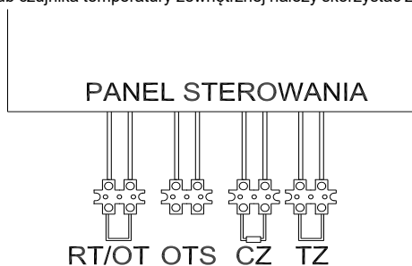
Rys.3.9.1 Płytkę sterownika
