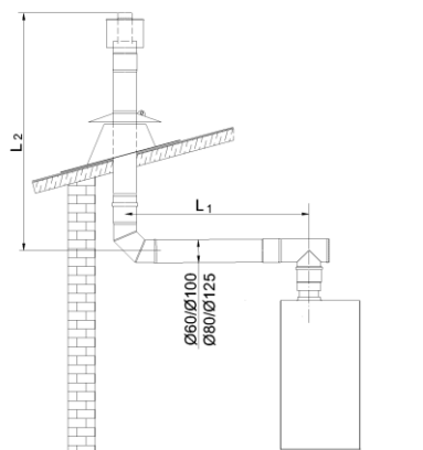
H = L_1 + L_2 + (1\text{m (strata na kolanku)}) + 1\text{m (strata na trójniku)} rys. 3.8.2.2
