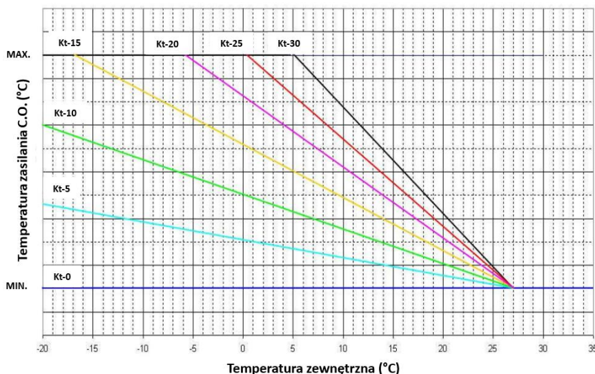
Rys.2.4.2.1 Wykres krzywych grzewczych
