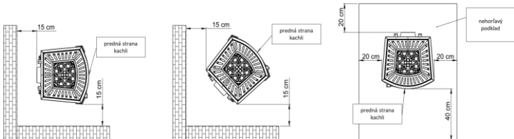
Obr. 2. Bezpečná vzdialenosť peci od nehorľavých častí.
