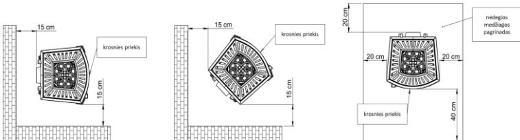
2. pv. Saugūs krosnies atstumai nuo nedegių dalių.
