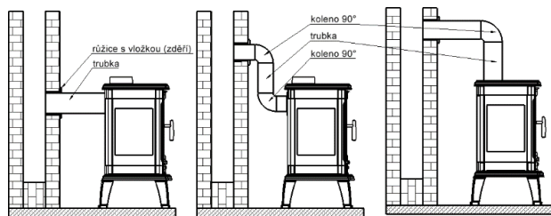
Obr. 3. Schéma zapojení kamen
