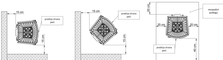
Crtež 2. Sigurne udaljenosti peći od nezapaljivih dijelova.
