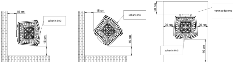
şek. 2. Ocağın yanıcı olmayan parçalara güvenli mesafeleri.
