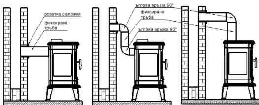
Фиг. 3. Схема за свързване на каминна печка
