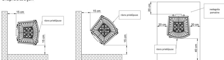
Att. 2. Droši plīts attālumi no nedegošām daļām.
