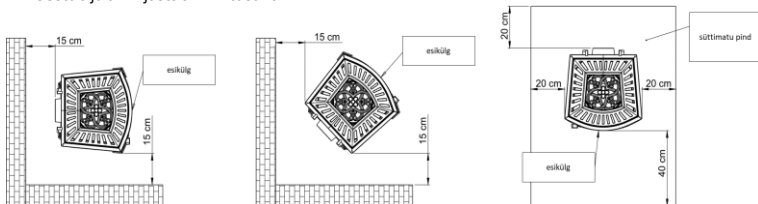
Joonis 2. Ahju ohutu kaugus mittesüttivatest osadest.
