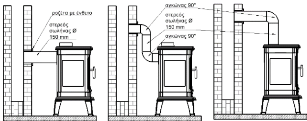
Σχ.3. Σχήμα σύνδεσης τζακιού
