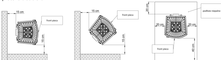
Rys.2. Bezpieczne odległości pieca od części niepalnych.
