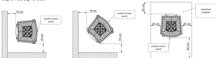
Obr. 3. Bezpečná vzdialenosť peči od nehorľavých častí.
