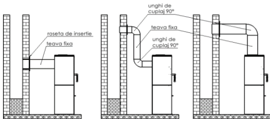
Fig.4. Schema de instalare a sobelor
