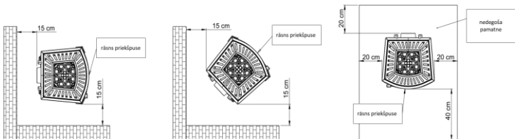
Att. 3. Droši plīts attālumī no nedegošām daļām.
