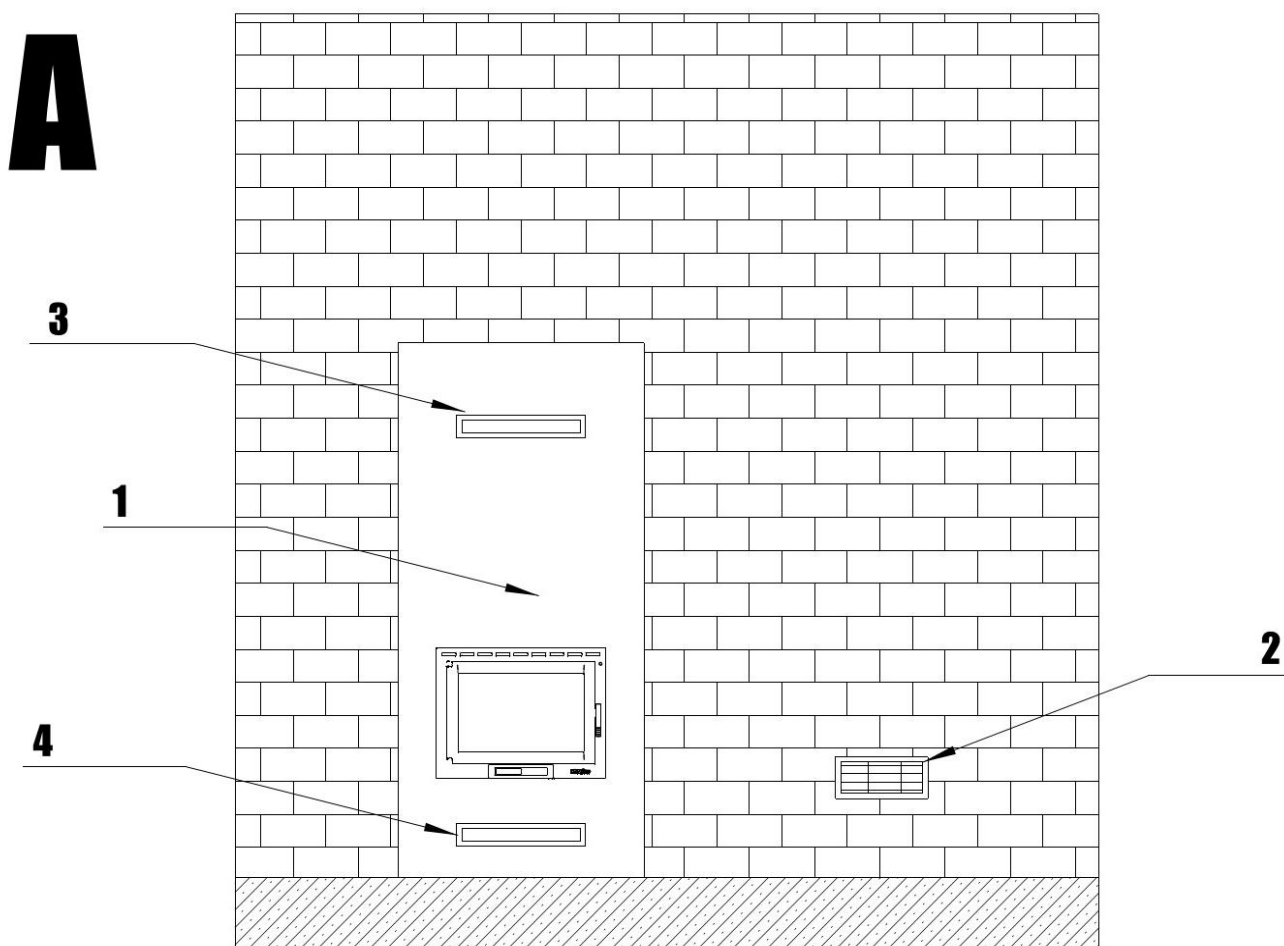
Rys. 3. [PL] Doprowadzenie powietrza/ [CZ] Přívod vzduchu/ [HU] Légbevezetés/ [SK] Prívod vzduchu/ [EN] Air supply/ [LT] Oro tiekimas/ [LV] Gaisa padeve/ [RU] Подача воздуха/ [EE] Õhuvarustus/ [GR] Παροχή αέρα/ [RO] Alimentarea cu aer/ [BG] Подаване на въздух/ [UA] Подача повітря/ [NL] Luchttoevoer/ [HR] Dovod zraka/ [TR] Havanın beslenmesi/ [PT] Aporte de ar/ [FR] Arrivée d'air/ [ES] Suministro de aire
