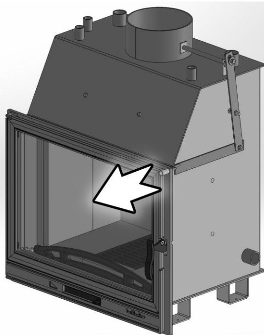
Rys. 6. [PL] Regulacja szybra/ [CZ] Nastavení dvířek/ [HU] Az üvegajtó állítása/ [SK] Nastavenie komínovej klapky/ [EN] Damper control/ [LT] Sklendės reguliavimas/ [LV] Aizbīdņa regulēšana/ [RU] Регулировка шибер/ [EE] Siibri reguleerimine/ [GR] Ρύθμιση κλαπέτου/ [RO] Ajustare sticlă/ [BG] Регулиране на клапата/ [UA] Регулювання заслінки/ [NL] Demper regeling/ [HR] Podešavanje zaklopke/ [TR] Damperin ayarı/ [PT] Regulação da comporta/ [FR] Réglage du clapet/ [ES] Regulación de la compuerta de tiro
