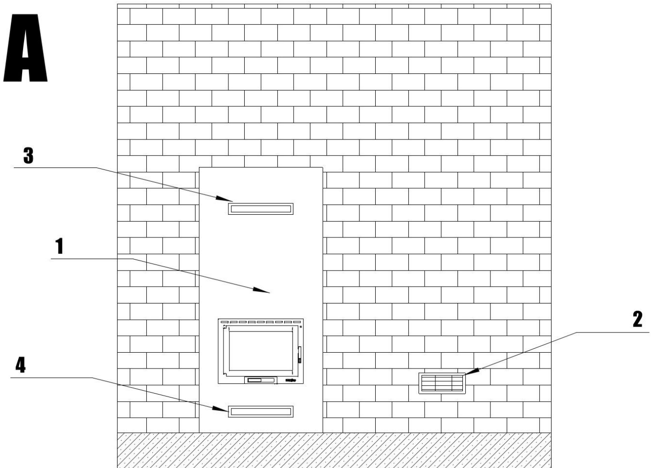
Rys. 3. [PL] Doprowadzenie powietrza/ [CZ] Přívod vzduchu/ [HU] Légbevezetés/ [SK] Prívod vzduchu/ [EN] Air supply/ [LT] Oro tiekimas/ [LV] Gaisa raideve/ [RU] Подача воздуха/ [EE] Õhuvarustus/ [GR] Παροχή αέρα/ [RO] Alimentarea cu aer/ [BG] Подаване на въздух/ [UA] Пoдaчa пoвiтpя/ [NL] Luchttoevoer/ [HR] Dовoд зpакa/ [TR] Havanın beslenmesi/ [PT] Aporte de ar/ [FR] Arrivée d'air/ [ES] Suministro de aire
