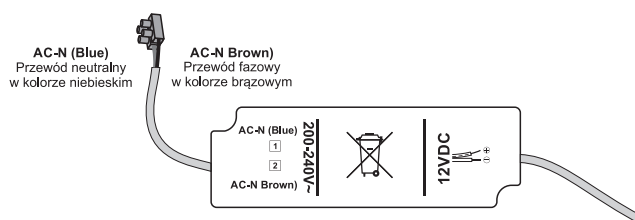
Rys 5. Schemat połączenia przewodów ze złączką
