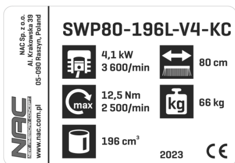
Tabliczka znamionowa
