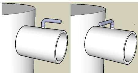
Otevřená poloha Uzavřená poloha Polohy ovládací páky pro nastavení hradítka (škrťací klapky spalin) v kouřovodu
