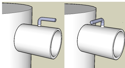
Открытое положение Закрытое положение Позиции положения ручки для регулирования шибер (дросселя выхлопов) в дымопроводе
