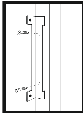
Zamknięcie do furtki
