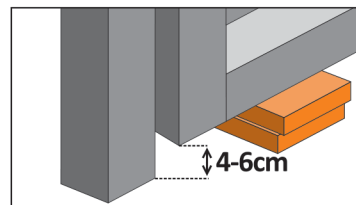
ODLEGŁOŚĆ SKRZYDŁA BRAMY I FURTKI OD PODŁOŻA
