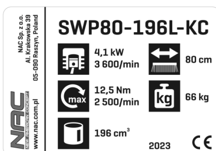
Tabliczka znamionowa
