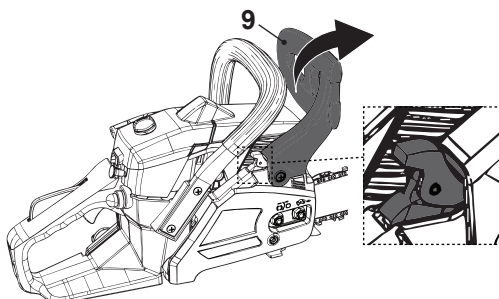
Rys. 23, włączanie hamulca łańcucha
