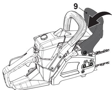
Rys.22, wyłączanie hamulca łańcucha
