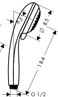
Crometta 85 Vario 28562000 / 27559005
